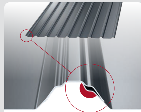
Kapilární profilování je dostupné v každé variantě profilu
