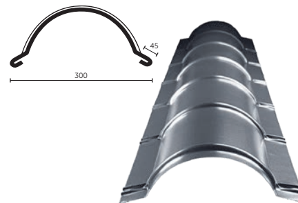
Hřebenáč pro rovný hřeben a pro hřeben nároží GS-30
